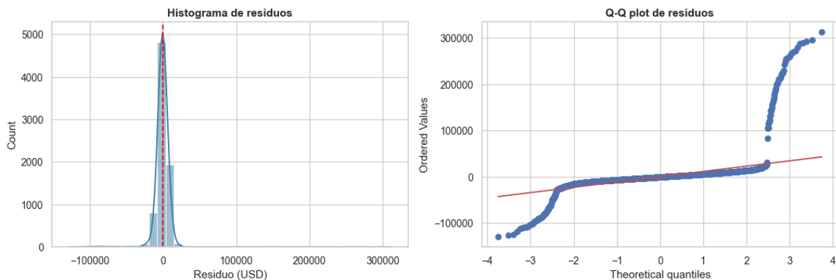
Figura 6. Histograma y Q-Q plot de los residuos del modelo.
